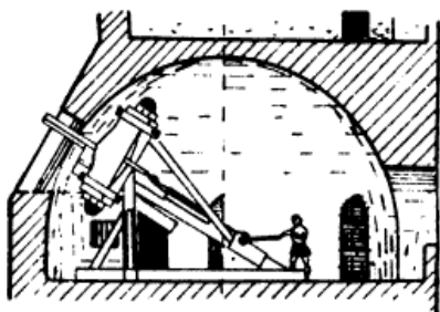
Изображение реконструкции расположения баллисты внутри башни древнеримской крепости I в. до н.э. – V в. н.э.
